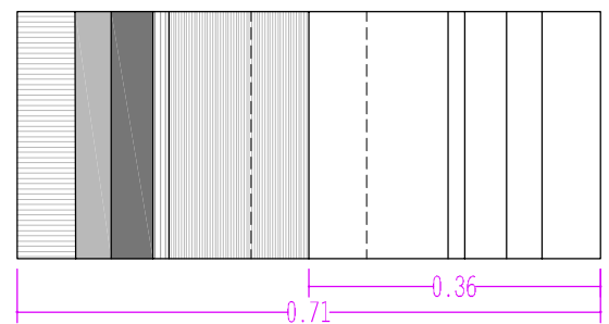
RICOSTRUZIONE DELLA SAGOMA DEI MERLI IN TESTA AL MURO D4 scala 1:10
